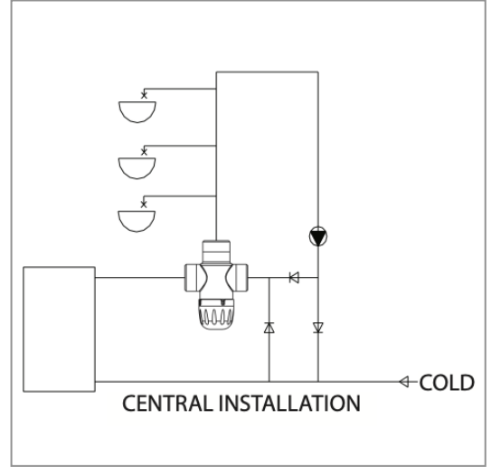
TMV tipik uygulama şeması
